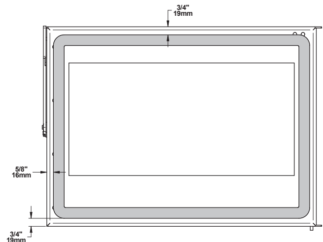
Figure 24: Remplacer le joint d'étanchéité de la vitre
