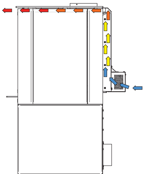
Figure 18: Circulation de l'air
