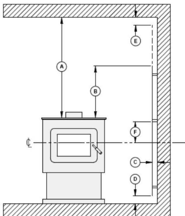
Figure 35: Dégagements pour l'écran de chaleur
