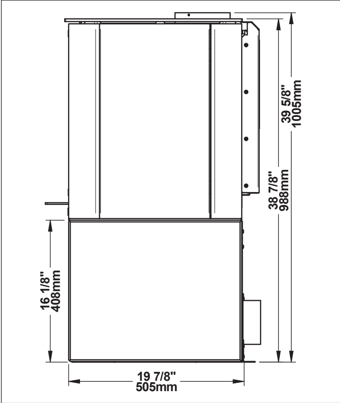
Figure 10: Vue de côté
