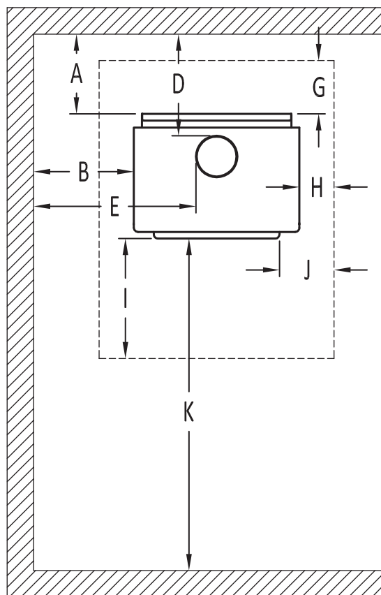
Figure 30: Développements - Dessus
