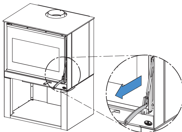
Figure 17: Tirer pour ouvrir
