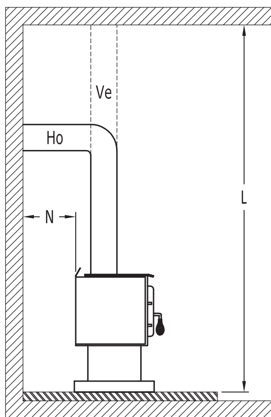
Figure 31: Développements - Côté
