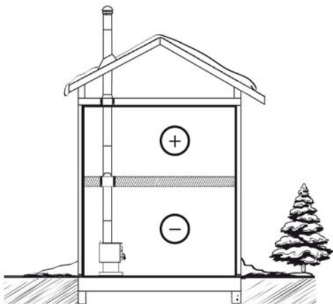
Figure 38: Bonne conception du système
