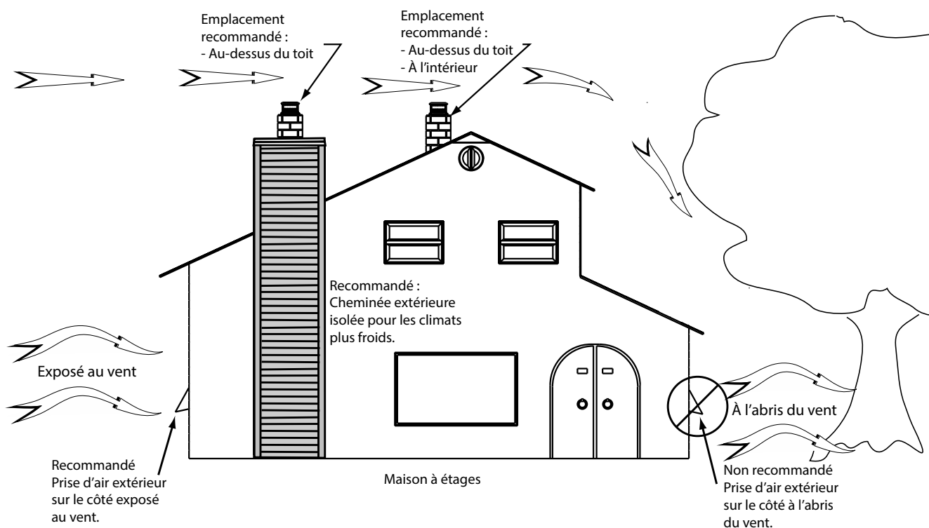
Figure 40: Apport d'air dans les maisons conventionnelles
