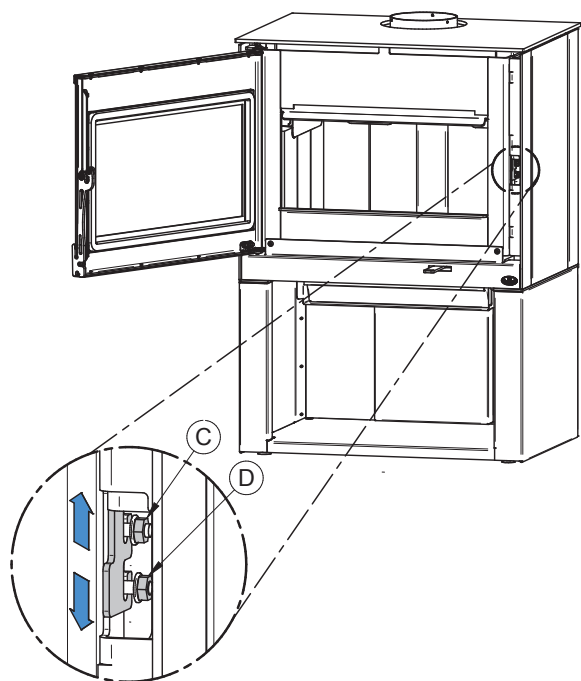
Figure 27: Ajustement de l'angle de la poignée
