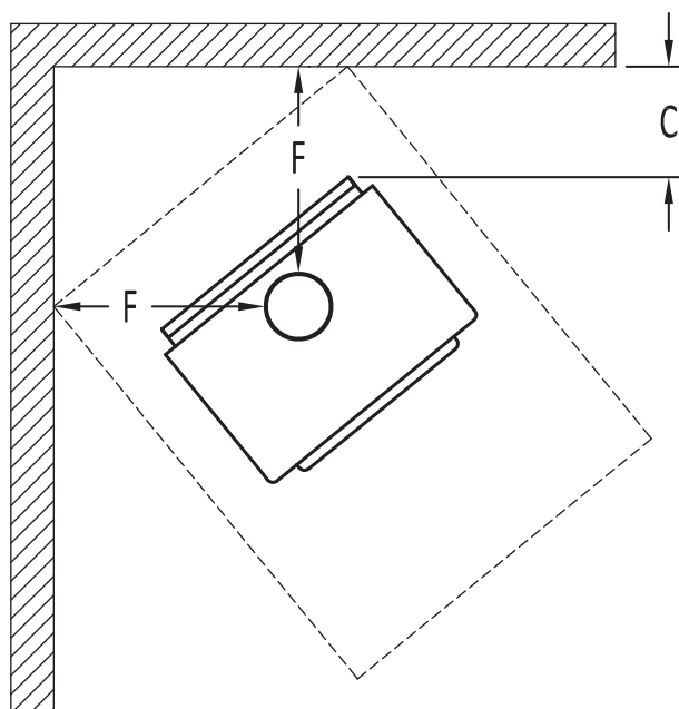
Figure 32: Développements - Coin
