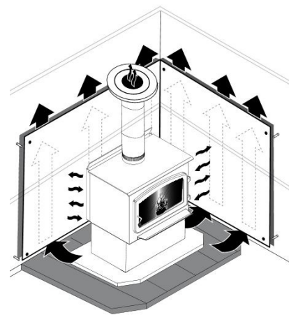
Figure 34: Écran de chaleur
