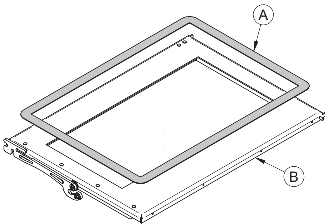
Figure 24: Remplacer le joint d'étanchéité de la vitre
