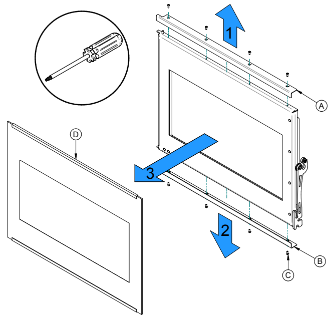
Figure 22: Remplacement la vitre
