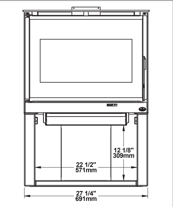
Figure 9: Vue de face
