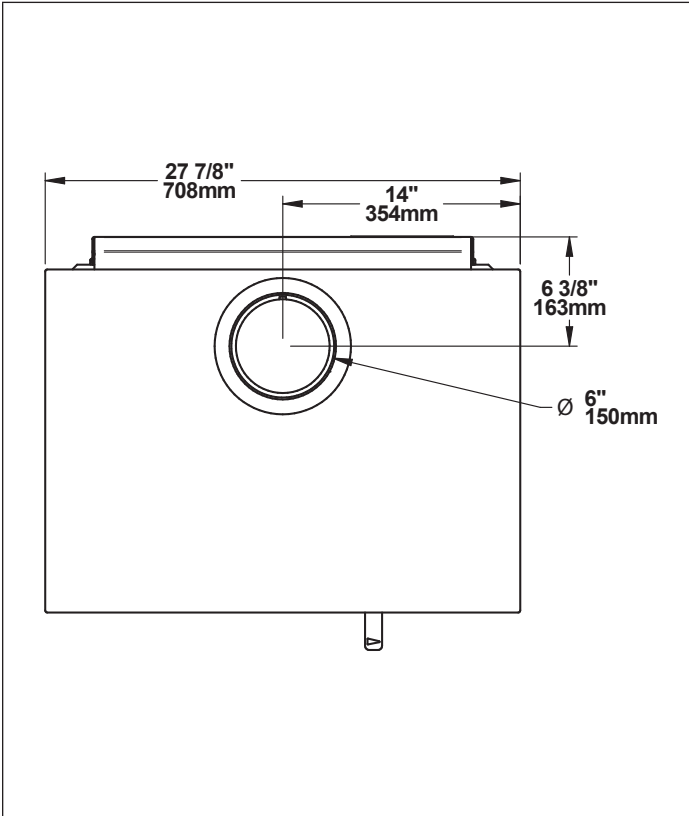
Figure 8: Vue de dessus
