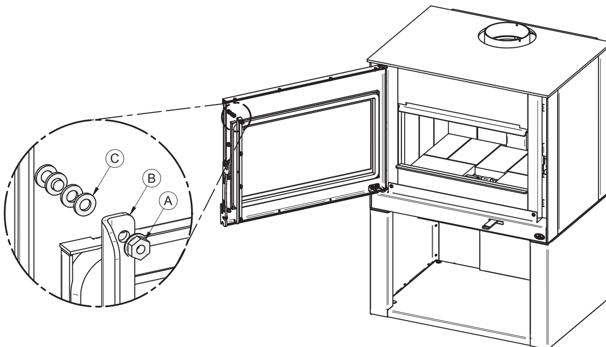
Figure 26: Ajustement de la porte avec l'équerre
