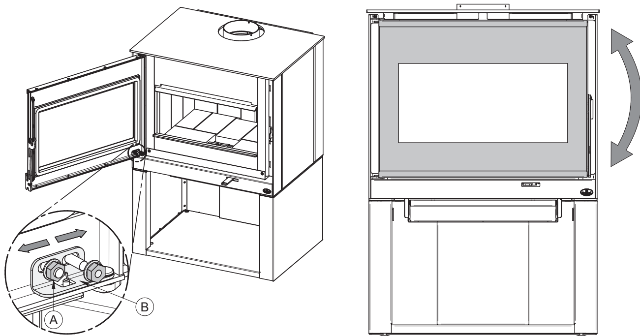
Figure 28: Ajustement de l'angle de la porte
