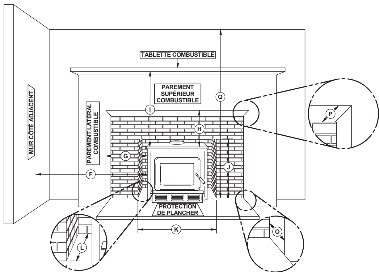
Figure 15: Ouverture de l’âtre et dégagements aux combustibles
