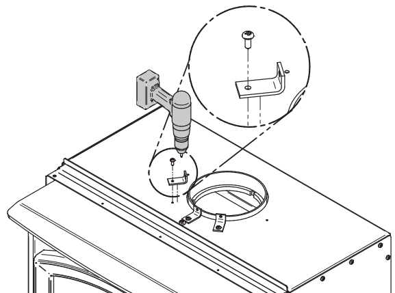
Figure 19: Installation des équerres
