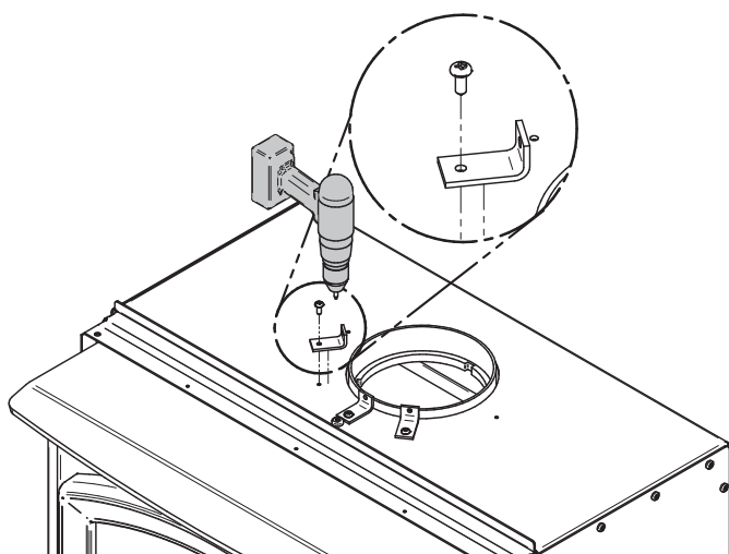
Figure 21: Installation des équerres
