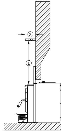
Figure 11: Dégagement de la tablette
