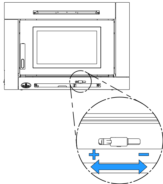
Figure 10: Contrôle de l'admission d'air
