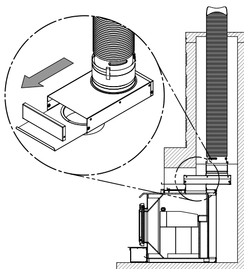
Figure 22: Adaptateur de déviation de gaine
